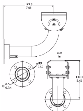
Короткий настенный кронштейн LTC 9215/00S для использования внутри помещений
