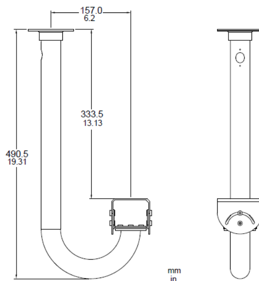
J-образный кронштейн со сквозной проводкой LTC 9219/01 для использования внутри помещений
