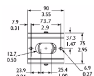
Настенный кронштейн LTC 9215/00 для использования вне помещений
