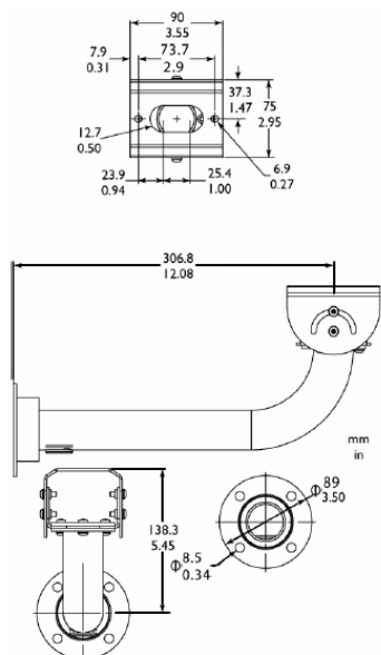
Настенный кронштейн LTC 9215/00 для использования вне помещений
