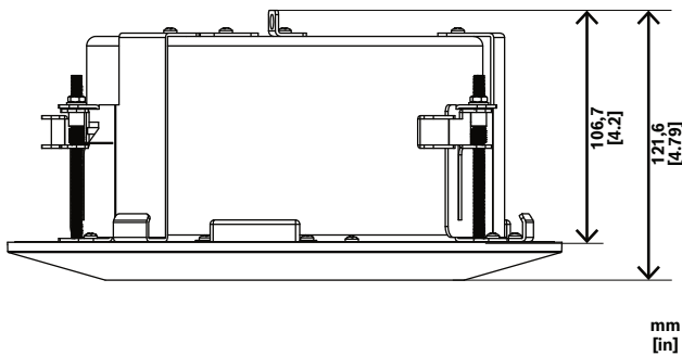
Fig. 2: NDA-8002-PLEN sin infrarrojos Dimensiones en mm (pulgadas)
