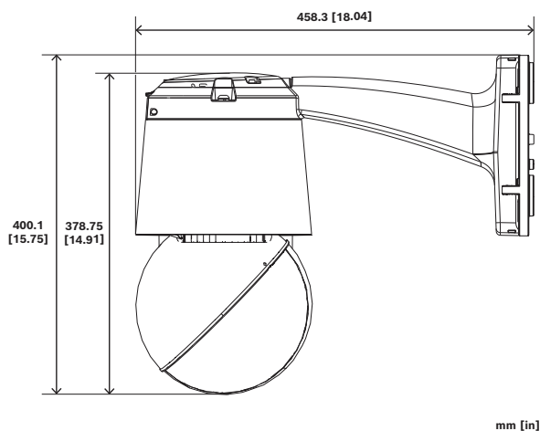
Рис. 1: Размеры камеры в мм (дюймах) при установке на NDA-7100-PEN | NDA-7100-PENF с NDA-PEND-WPLATE (вид сбоку)
