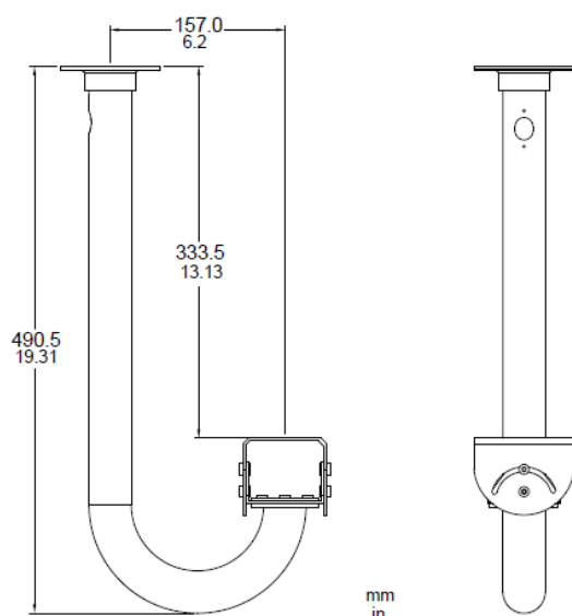
LTC 9215/00S Korte wandbeugel voor gebruik binnenshuis
