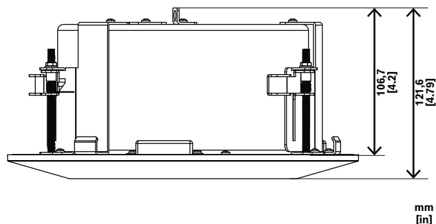
Afb. 2: NDA-8002-PLEN zonder IR Afmetingen in mm (inch)
