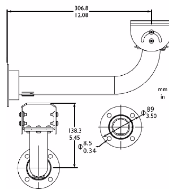
LTC 9215/00 Support mural pour l'extérieur
