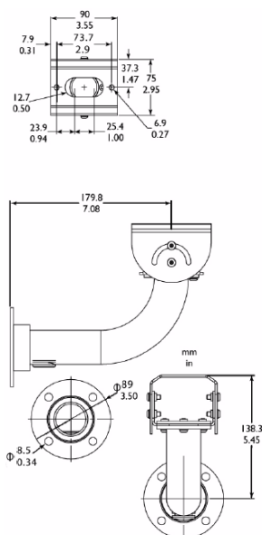
LTC 9215/00S Support mural court pour l'intérieur
