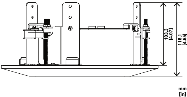
Fig. 2: NDA-8002-IC non IR Dimensions en mm (pouces)
