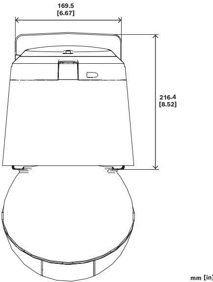
Fig. 2: Dimensiones en mm (pulg.) de la cámara en el dispositivo NDA-7100-PEN | NDA-7100-PENF (vista frontal)
