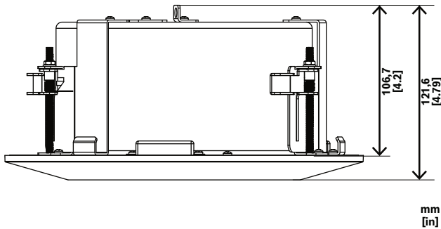
Fig. 2: NDA-8002-PLEN Non-IR Dimensions en mm (pouces)
