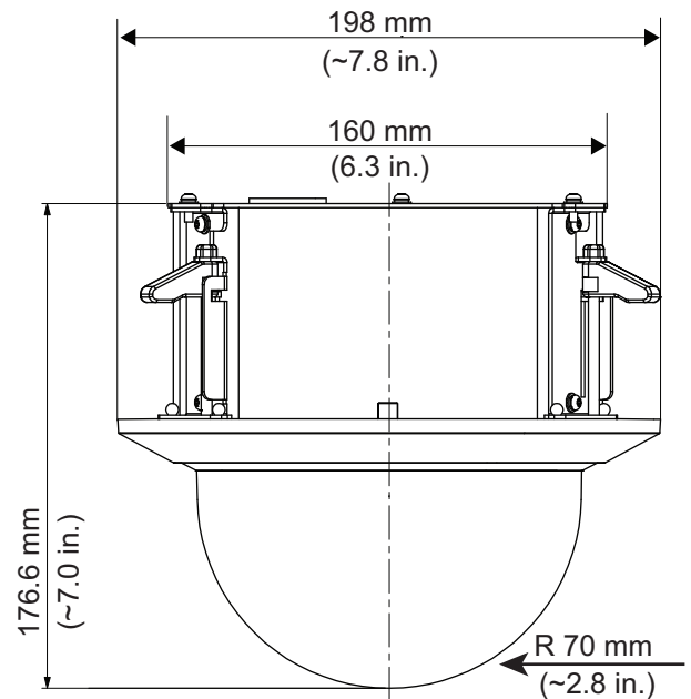
圖 1: 天花板掛架機型 尺寸，單位為公釐 (英吋)
